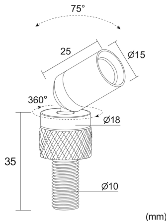
Testa Ø 15 × 25 mm · base Ø 18 · gambo Ø 10 × 35 mm
